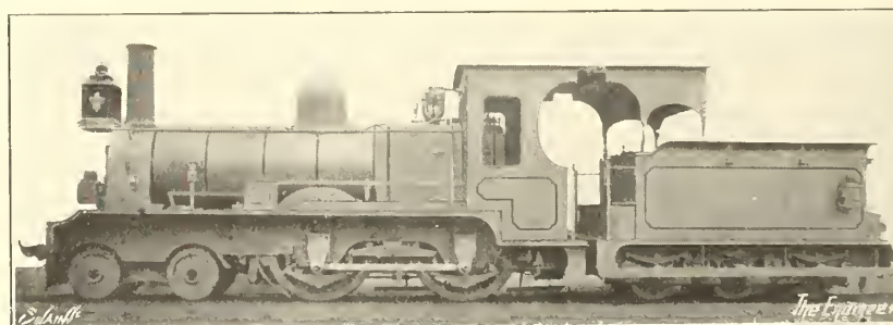
FIG. 395—METRE GAUGE ENGINE FOR THE RAJPUTANA-MALWA RLY.—DÜBS & CO., 1880
