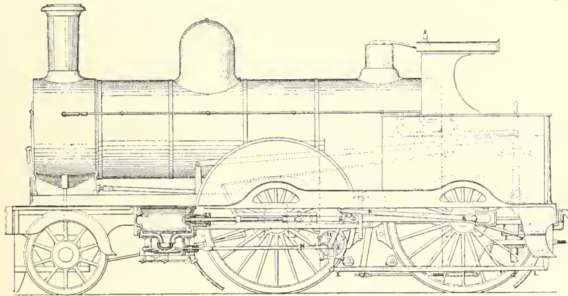
FIG. 307—F. W. WEBB'S L. & N.W.R. COMPOUND, 1882-83
