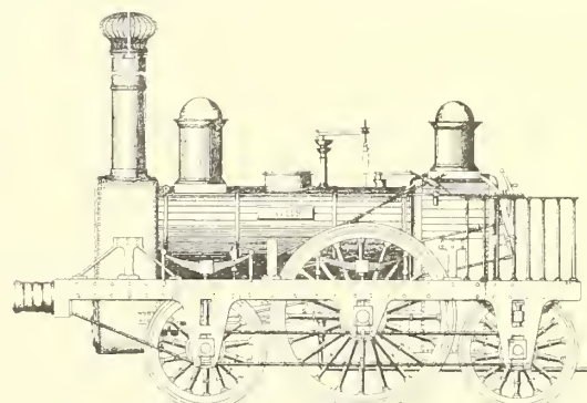
FIG. 31—TAYLEUR & CO. TYPE 2-2-2 ENGINE
